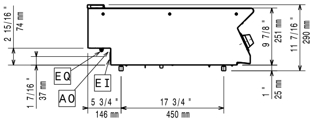
Oldalnézet
